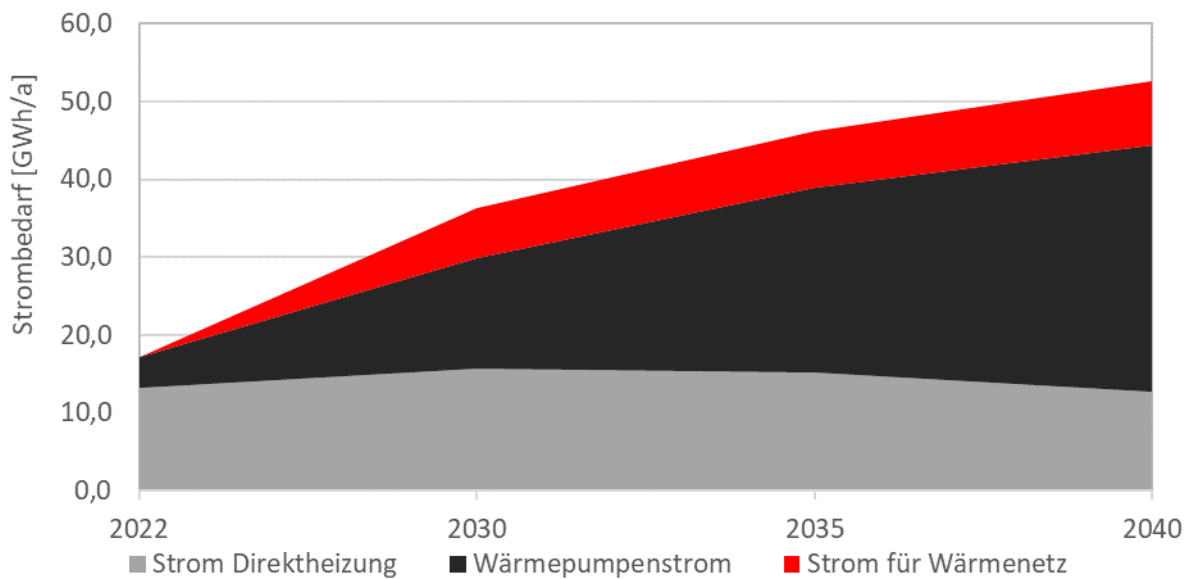
Abbildung 72: Strombedarfsentwicklung für die Wärmeversorgung
