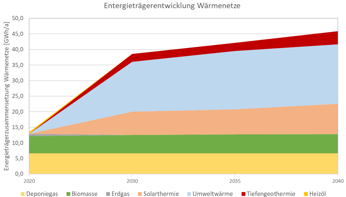
Abbildung 66: Energieträgerentwicklung der Wärmenetze im Konvoigebiet
