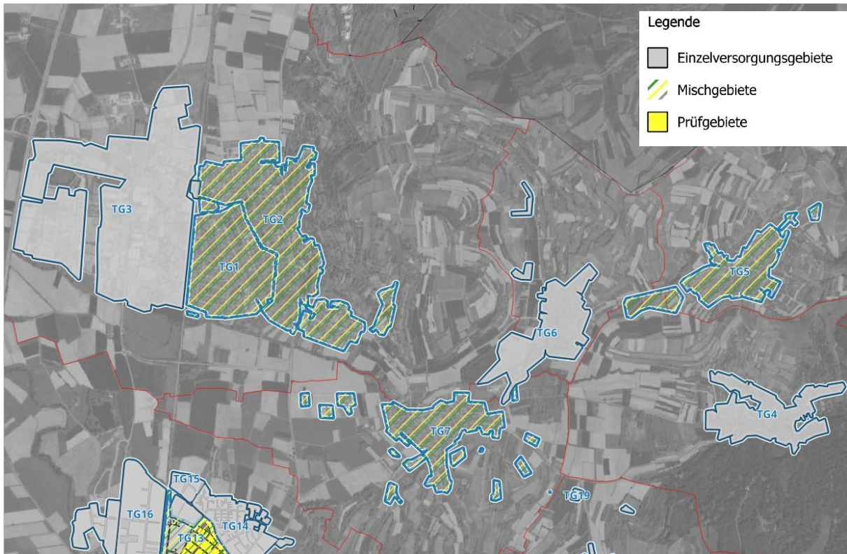
Abbildung 74: Versorgungslösungen je Teilgebiet - Herbolzheim
