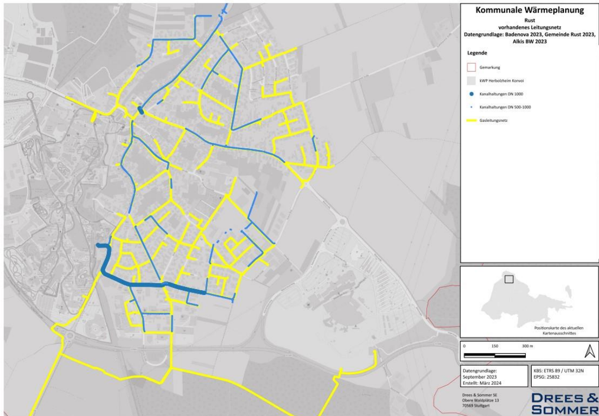
Abbildung 53: Leitungsnetze Rust
