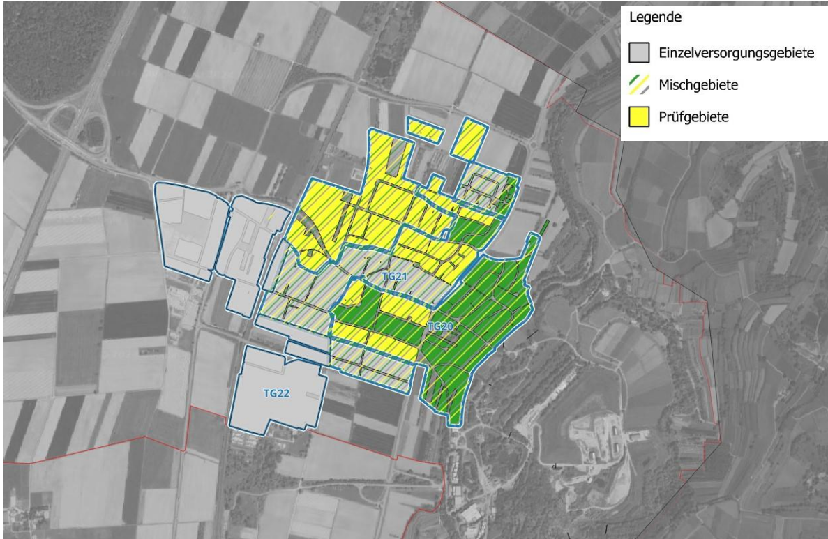
Abbildung 76: Versorgungslösungen je Teilgebiet - Ringsheim
